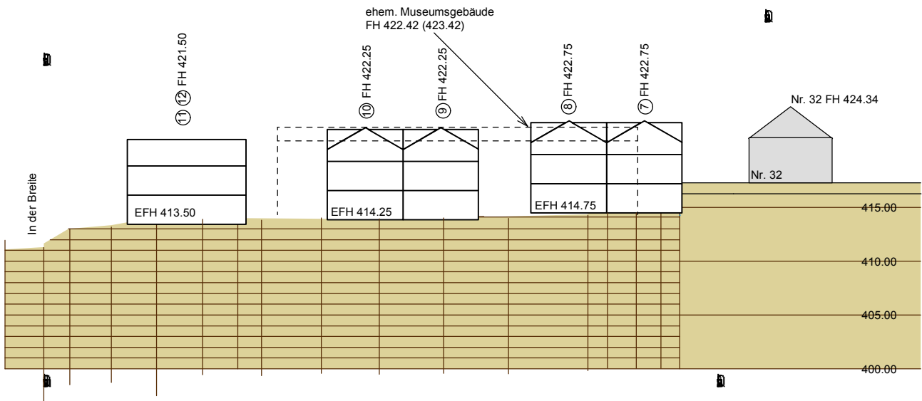
Längsschnitt Nord – Süd Schnitt 4: östl. Grundstücksbereich Blickrichtung West
