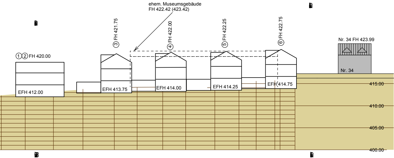
Längsschnitt Nord – Süd Schnitt 3: westl. Grundstücksbereich Blickrichtung West
