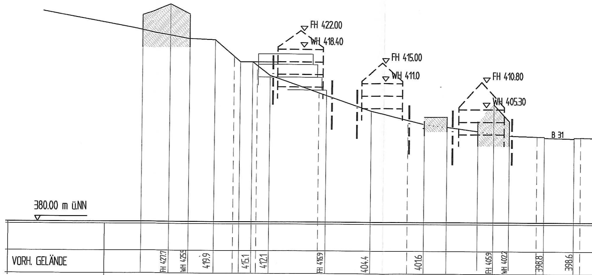
SCHEMASCHNITT A-A
