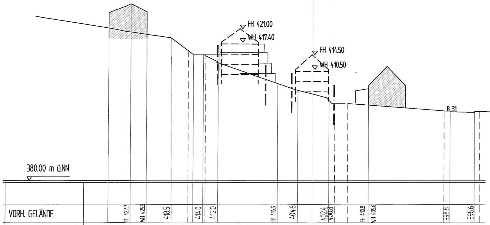
SCHEMASCHNITT B-B
